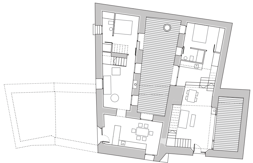
PLANTA BAJA
