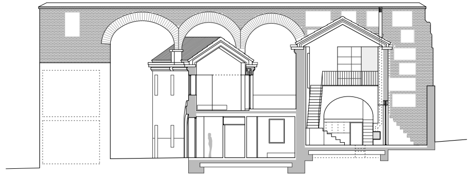
SECCIÓN S1
