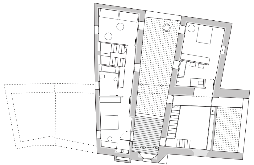
PLANTA NIVEL 1
