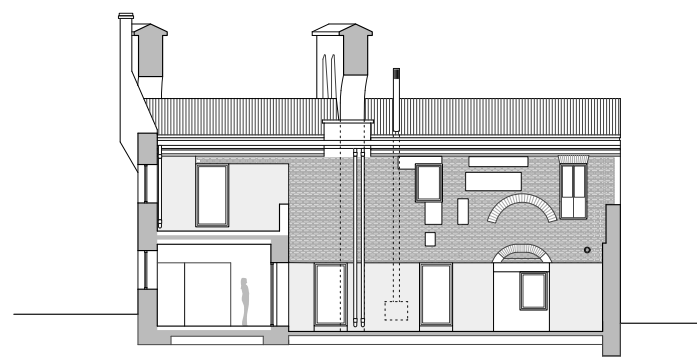
SECCIÓN S3
