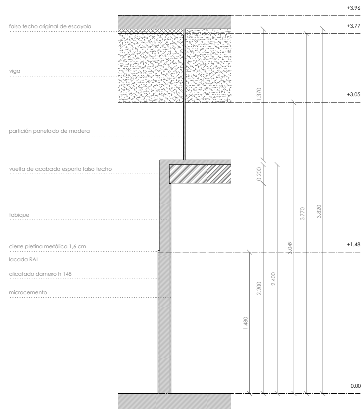
DETALLE 01 PARED COCINA | BAÑO 1/20 A1 1/40 A3
