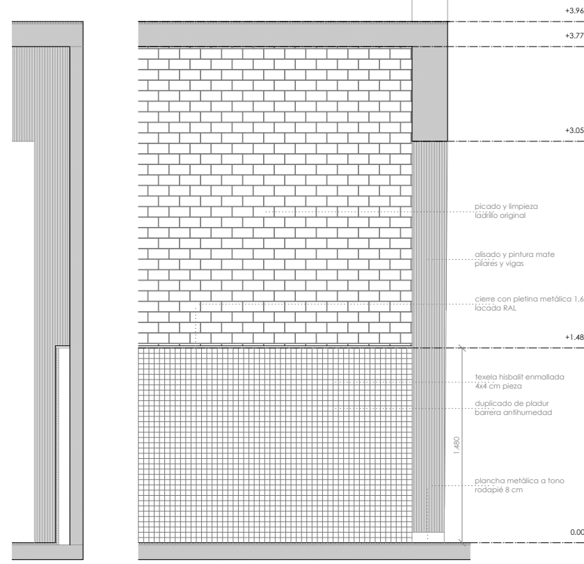
DETALLE 02 PARED TIPO 1/20 A1 1/40 A3
