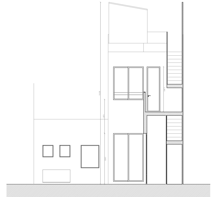
SECCIÓN a-a' ALZADO 03
