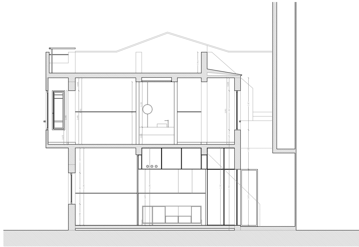
SECCIÓN VIVIENDA b-b'
