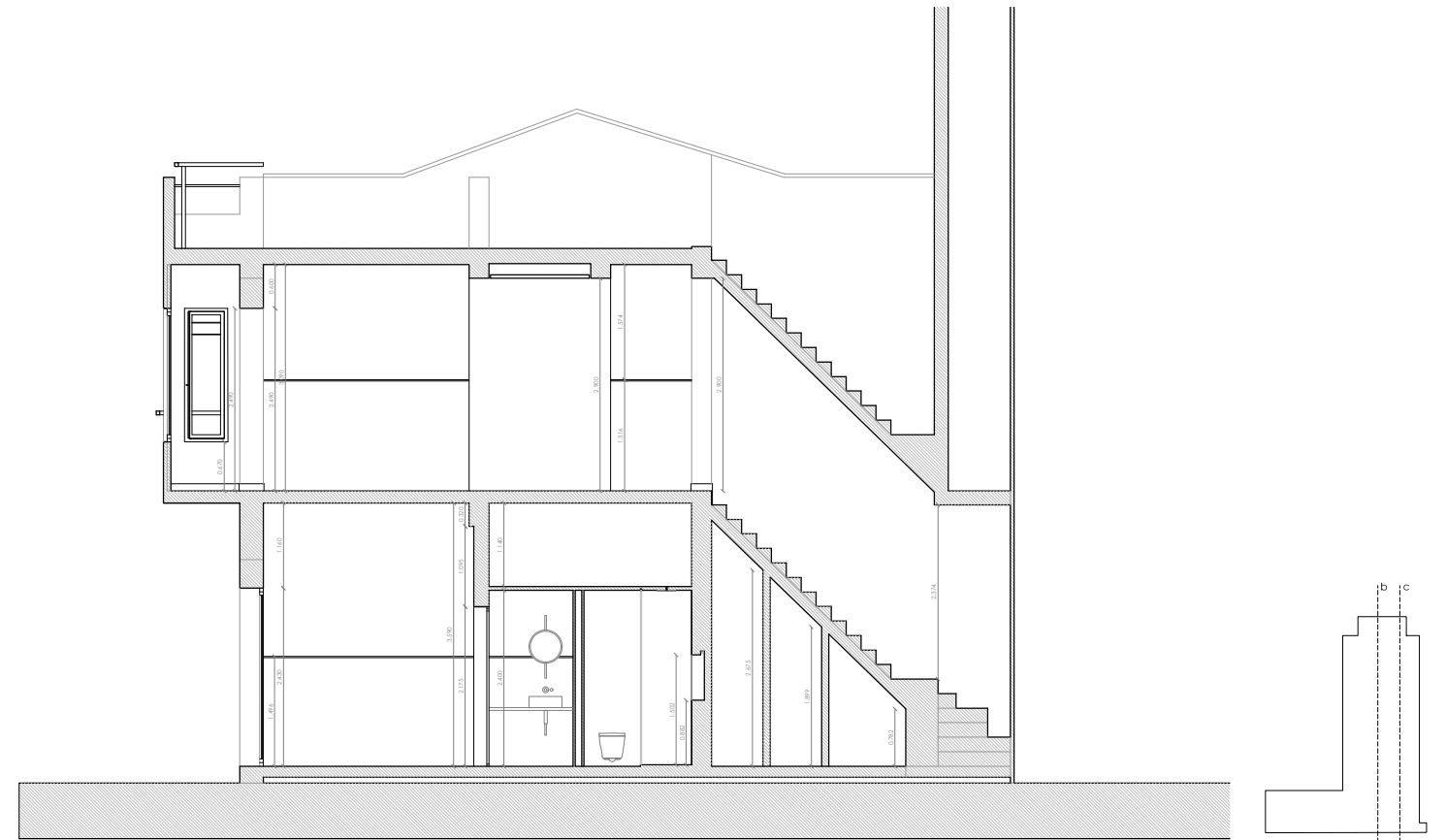
SECCIÓN VIVIENDA c-c'
