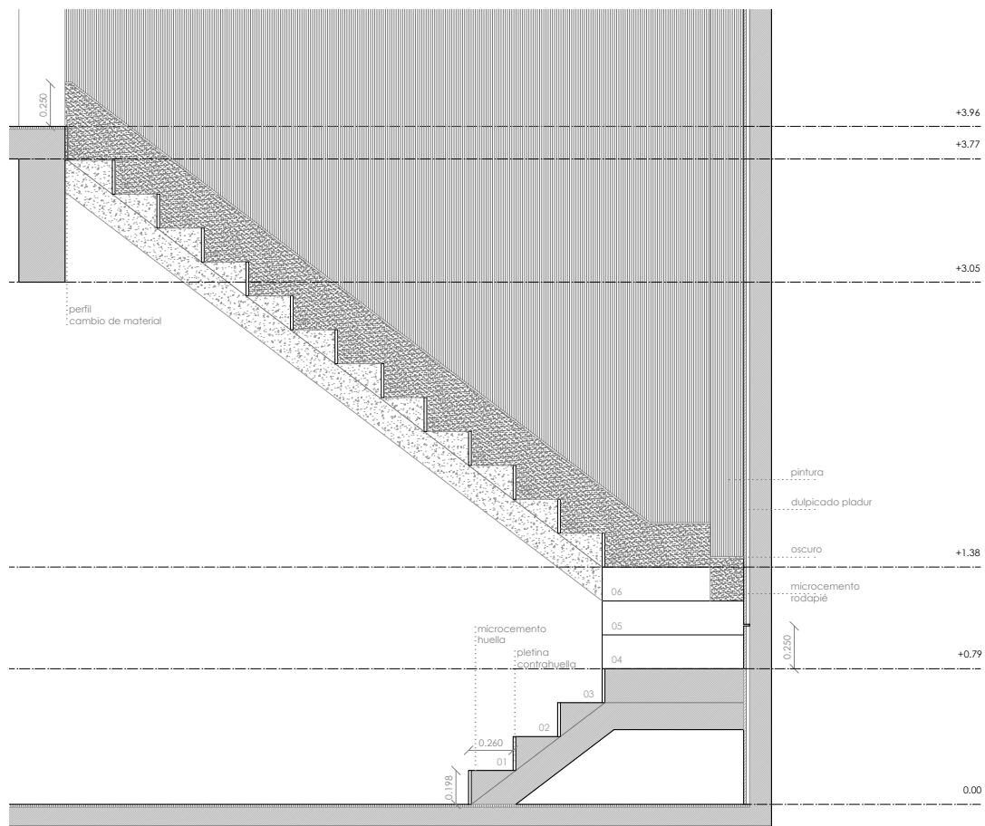
DETALLE 03 ESCALERA 1/20 A1 1/40 A3
