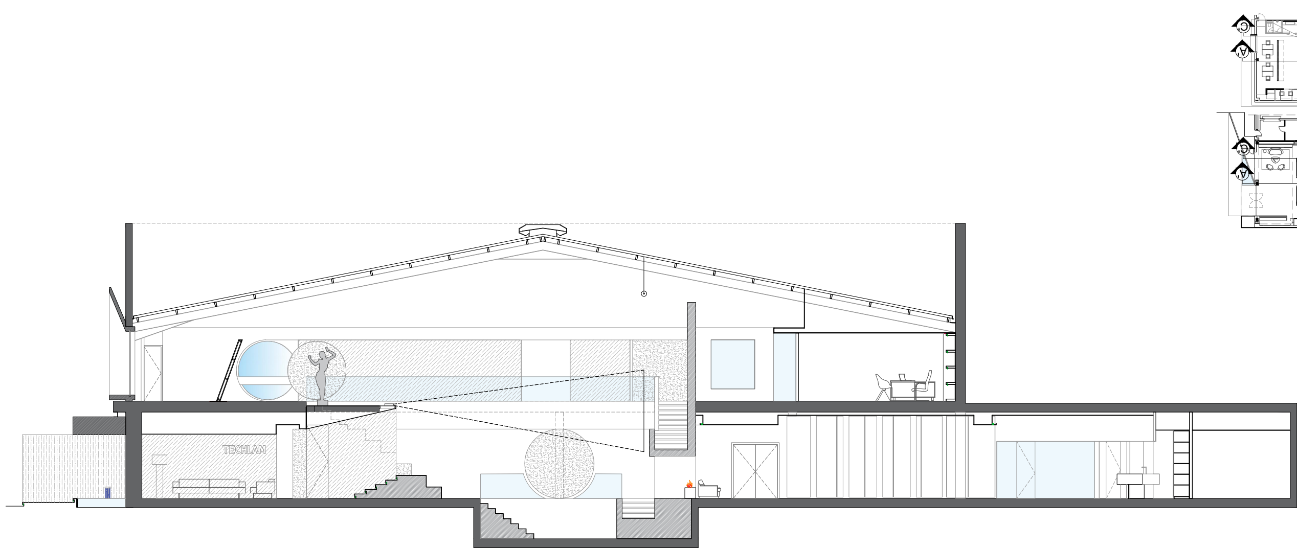
SECCIÓN AA'
