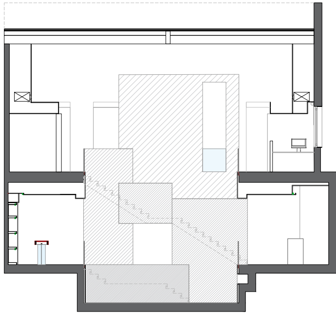
SECCIÓN EE'
