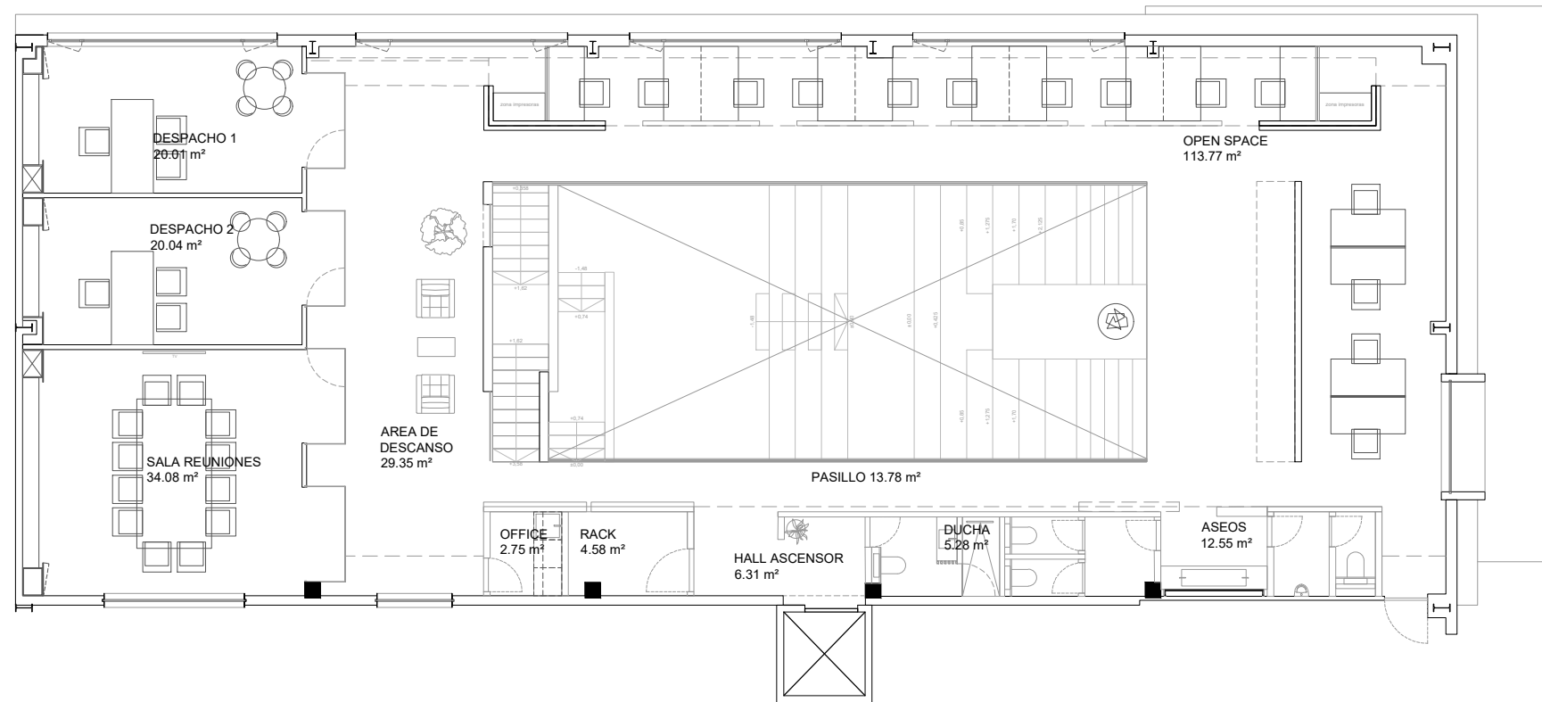
ESTADO REFORMADO PLANTA ALTA
