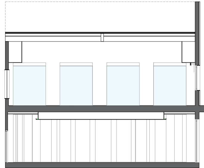
SECCIÓN FF'
